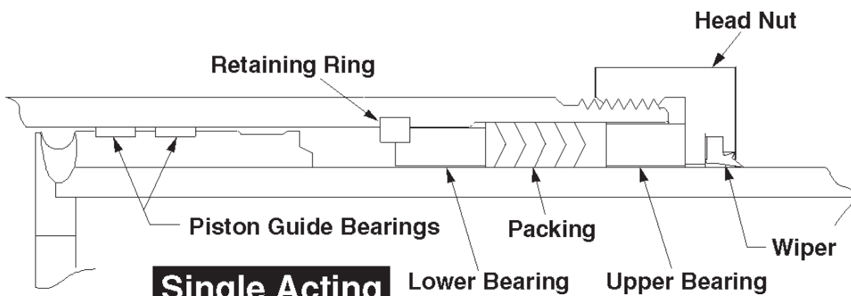
Hyco 30000
